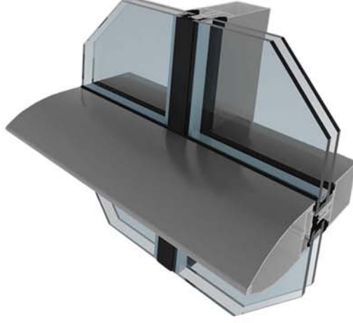
YKC-50 YARI KAPAKLI CEPHE SİSTEMİ (semi frame facade system)
