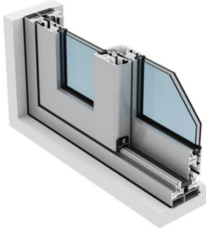
ISI-SH120 KALDIR & SÜR SİSTEMİ (lift & slide system)
