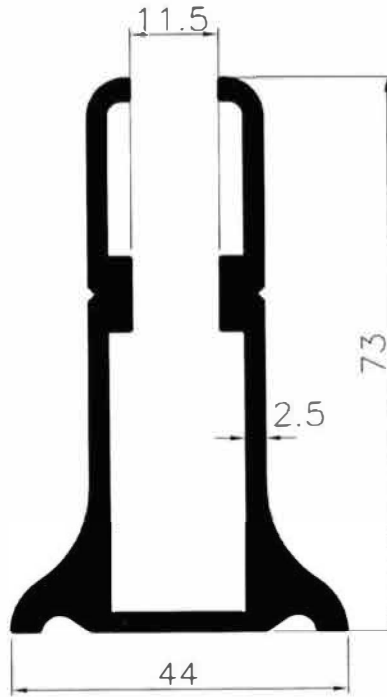
6028 1.724 Kg/m
