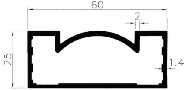
8074 0.903 Kg/m
