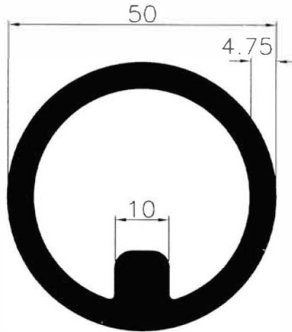
6836 2.081 Kg/m
