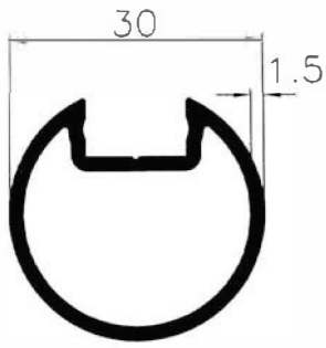
6695 0.411 Kg/m
