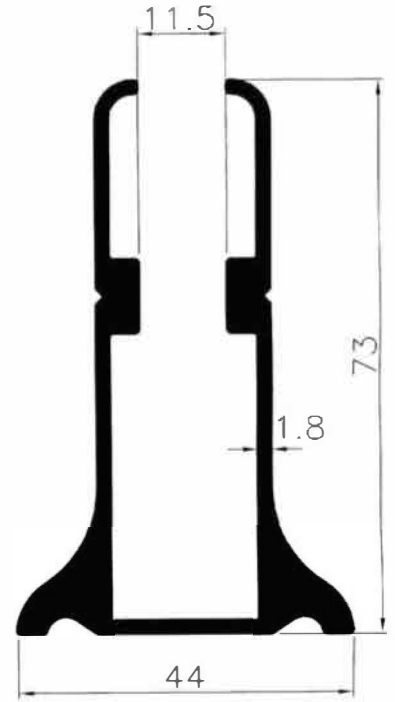
7863 1.450 Kg/m
