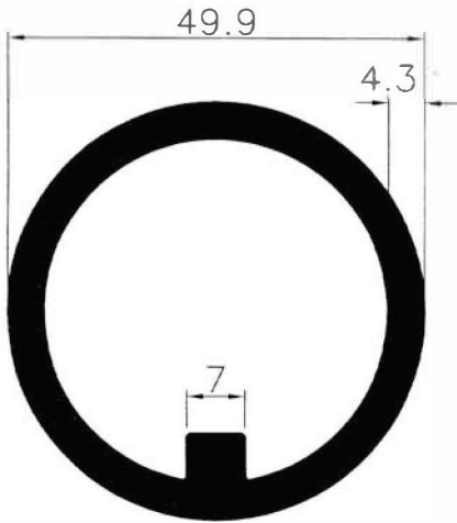
7917 1.775 Kg/m
