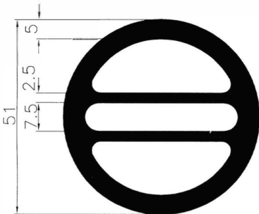
5161 2.574 Kg/m
