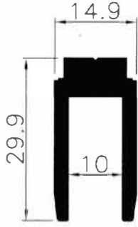
3044 0.535 Kg/m
