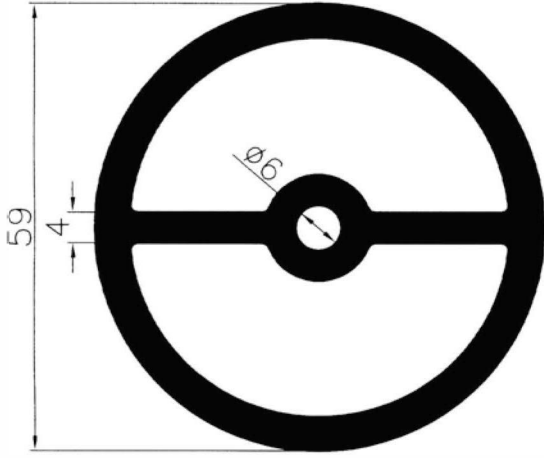
5159 2.814 Kg/m
