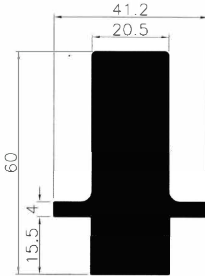
7991 3.575 Kg/m
