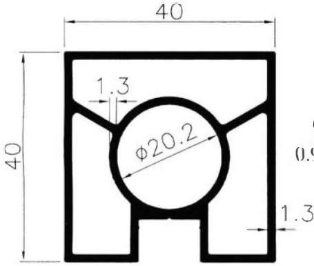
8072 0.892 Kg/m
