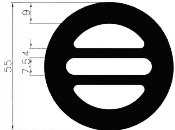
7131 4.329 Kg/m
