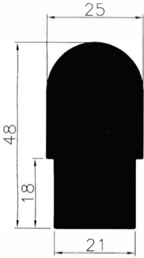
7990 2.864 Kg/m
