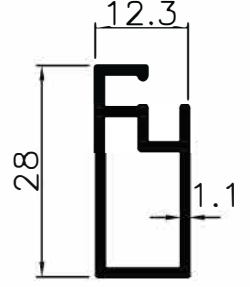
7458 ●.244 Kg/m
