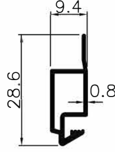
8137 ●.152 Kg/m
