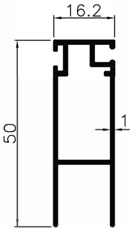
7451 ●.389 Kg/m
