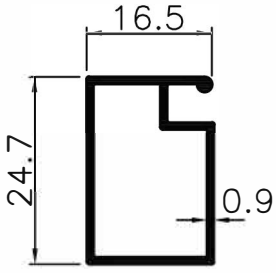
5965 ●.212 Kg/m
