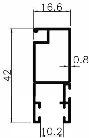
7450 ●.389 Kg/m
