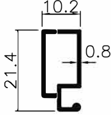
6056 ●.138 Kg/m
