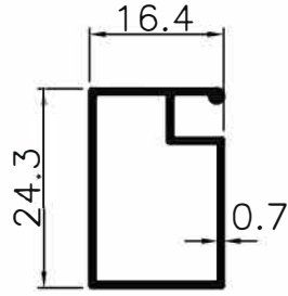
8063 ●.164 Kg/m
