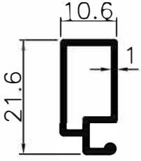
2119 ●.170 Kg/m
