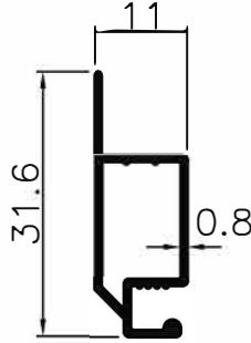
7541 ●.167 Kg/m
