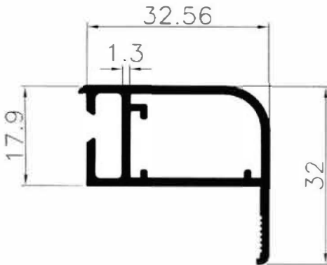
2763 0.437 Kg/m
