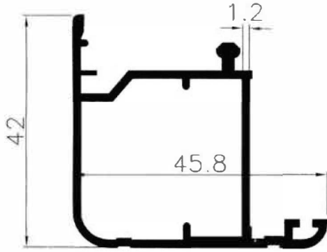
3619 0.592 Kg/m
