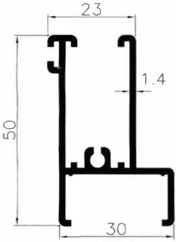
1901 0.613 Kg/m
