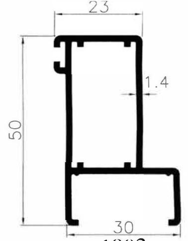
1903 0.608 Kg/m
