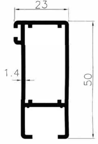
1900 0.538 Kg/m
